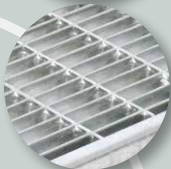
Caillebotis 30 x 10 Acier galvanisé
